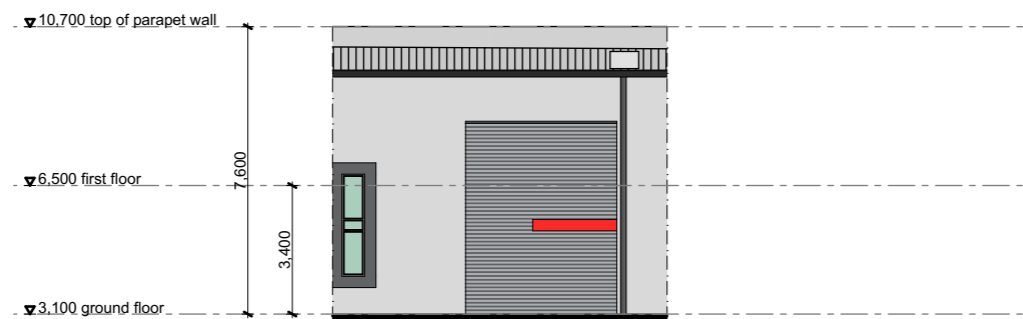
unit 221 elevation B
