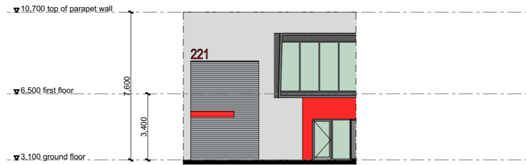
unit 221 elevation A
